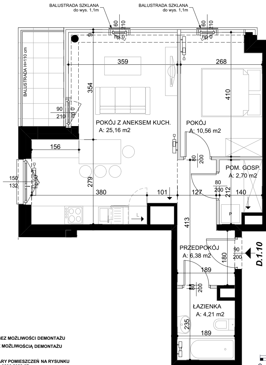
BUDYNEK MIESZKALNY WIELODZINNY Z USŁUGAMI W PARTERZE I GARAŻEM PODZIEMNYM
